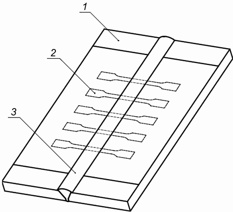
1 — краевая зона; 2 — расположение образцов; 3 — сварной шов
