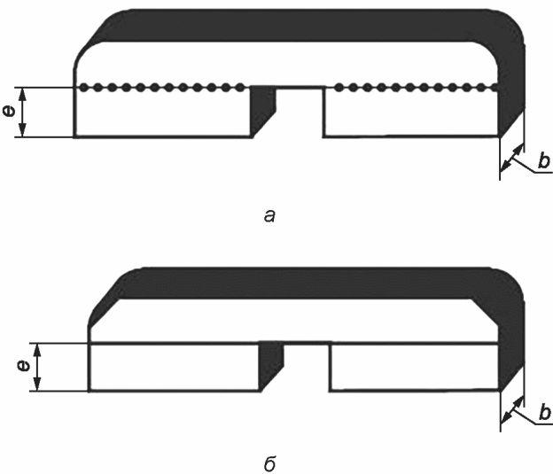
а — образец, выполненный сваркой ЗН; б — образец, выполненный сваркой НИр; b — ширина образца; е — толщина стенки трубы
