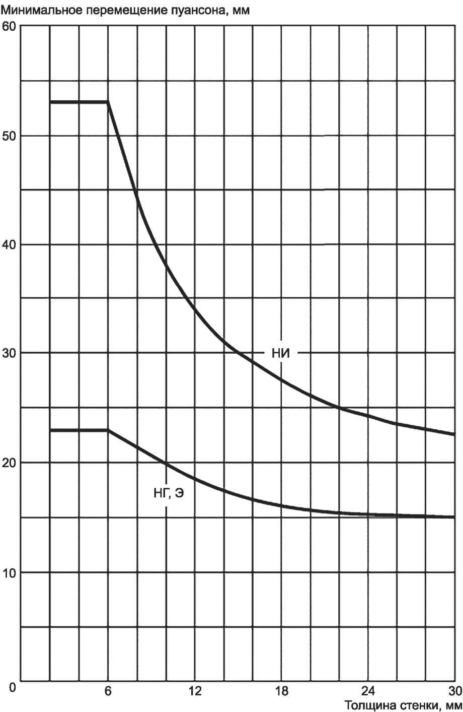
Рисунок Б.9 — Минимальное перемещение пуансона для ПП-Р (тип 3) в зависимости от толщины для разных методов сварки (верхняя кривая — для сварки НИ, нижняя — для сварки НГ и Э)
