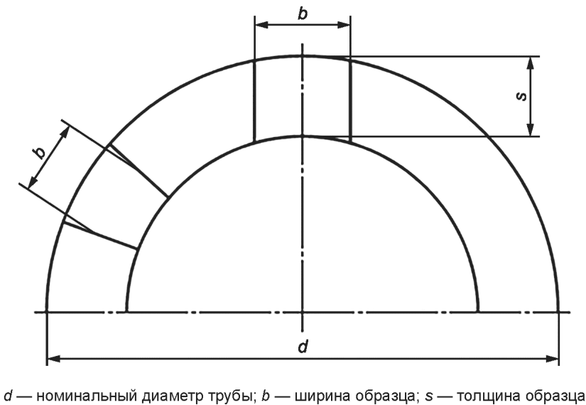
Рисунок 10 — Способы вырезания образцов из трубы
