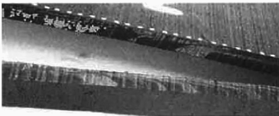
Рисунок В.8 — Образец ПЭ с гладкой поверхностью разрушения
