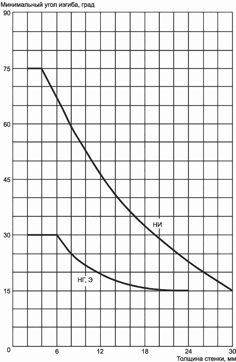
Рисунок Б.5 — Минимальный угол изгиба для НПВХ в зависимости от толщины для разных методов сварки (верхняя кривая — для сварки НИ, нижняя — для сварки НГ и Э)
