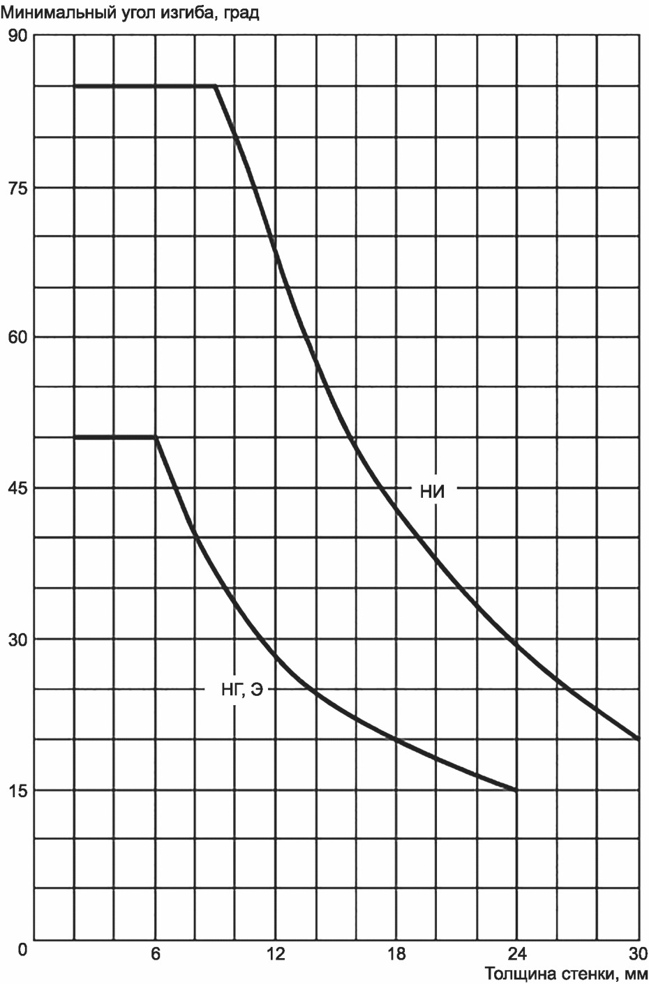
Рисунок Б.6 — Минимальный угол изгиба для УПВХ в зависимости от толщины для разных методов сварки (верхняя кривая — для сварки HI, нижняя — для HG и Z)
