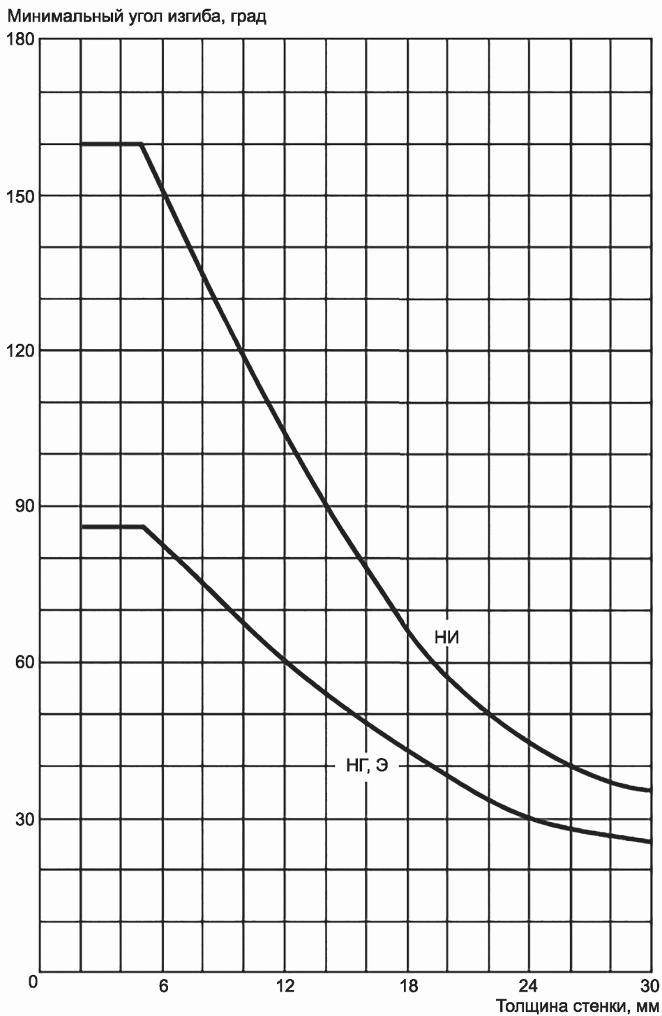
Рисунок Б.3 — Минимальный угол изгиба для ПП-Р (тип 3) в зависимости от толщины для разных методов сварки (верхняя кривая — для сварки НИ, нижняя — для сварки НГ и Э)
