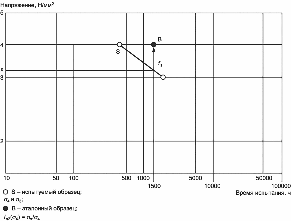
Рисунок 7 — Схема определения коэффициента f_s при длительных испытаниях на ползучесть с учетом одного испытательного напряжения образца из того же изделия без сварного соединения
