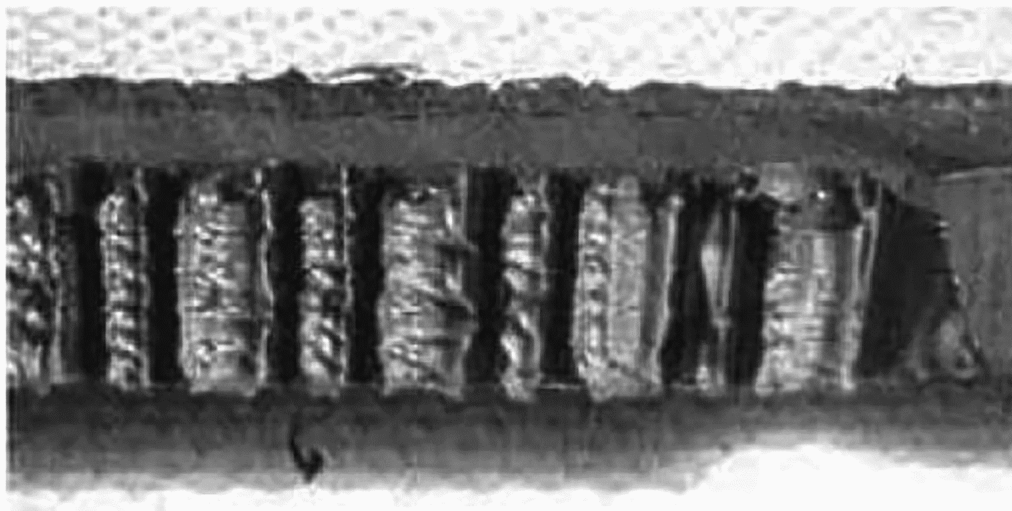
Рисунок В.7 — Образец ПЭ с пластической поверхностью разрушения
