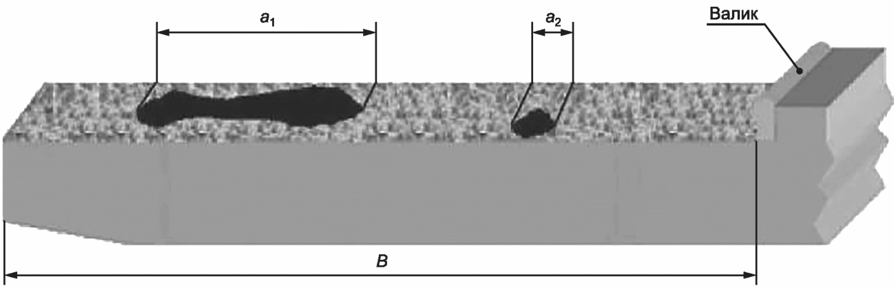
B — длина зоны сварки; a_1, a_2 — примеры дефектов
