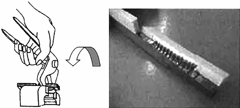
Рисунок В.6 — Испытание на радиальное расслаивание для соединений, выполненных сваркой ЗН и НИр
