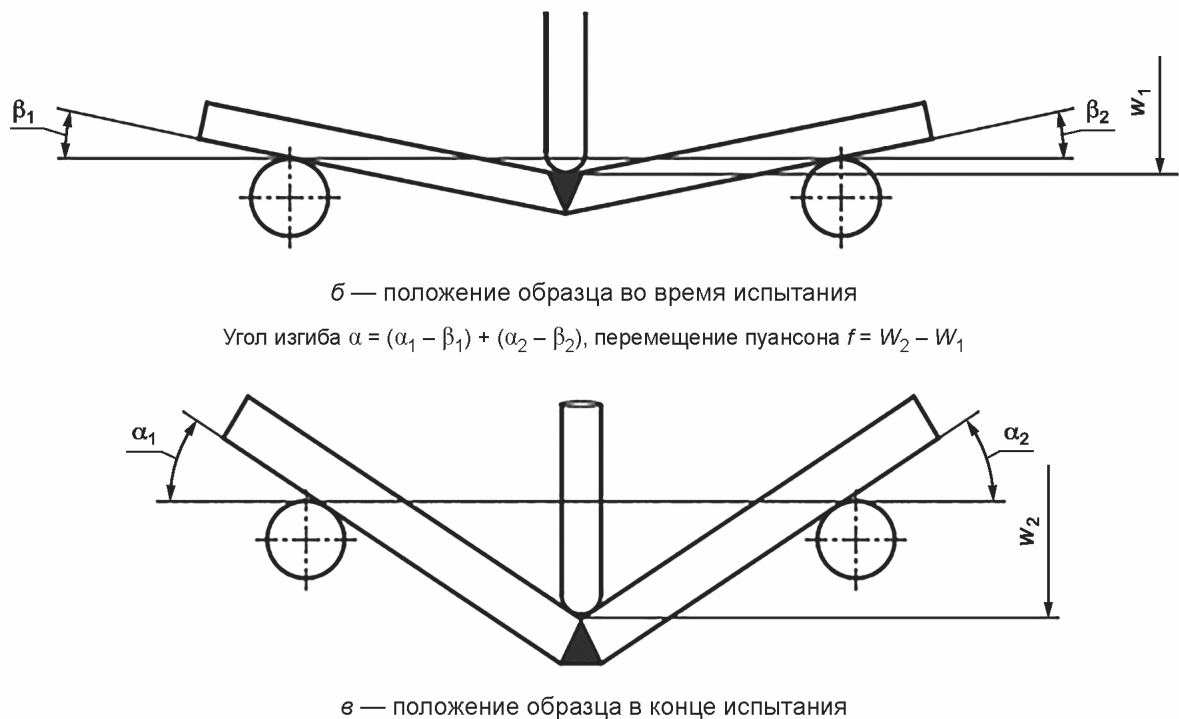
Рисунок 11 — Схематическое изображение процесса определения угла изгиба и перемещения пуансона
