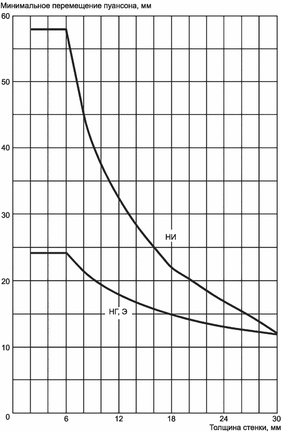
Рисунок Б.7 — Минимальное перемещение пуансона для ПЭ в зависимости от толщины для разных методов сварки (верхняя кривая — для сварки НИ, нижняя — для НГ и Э)
