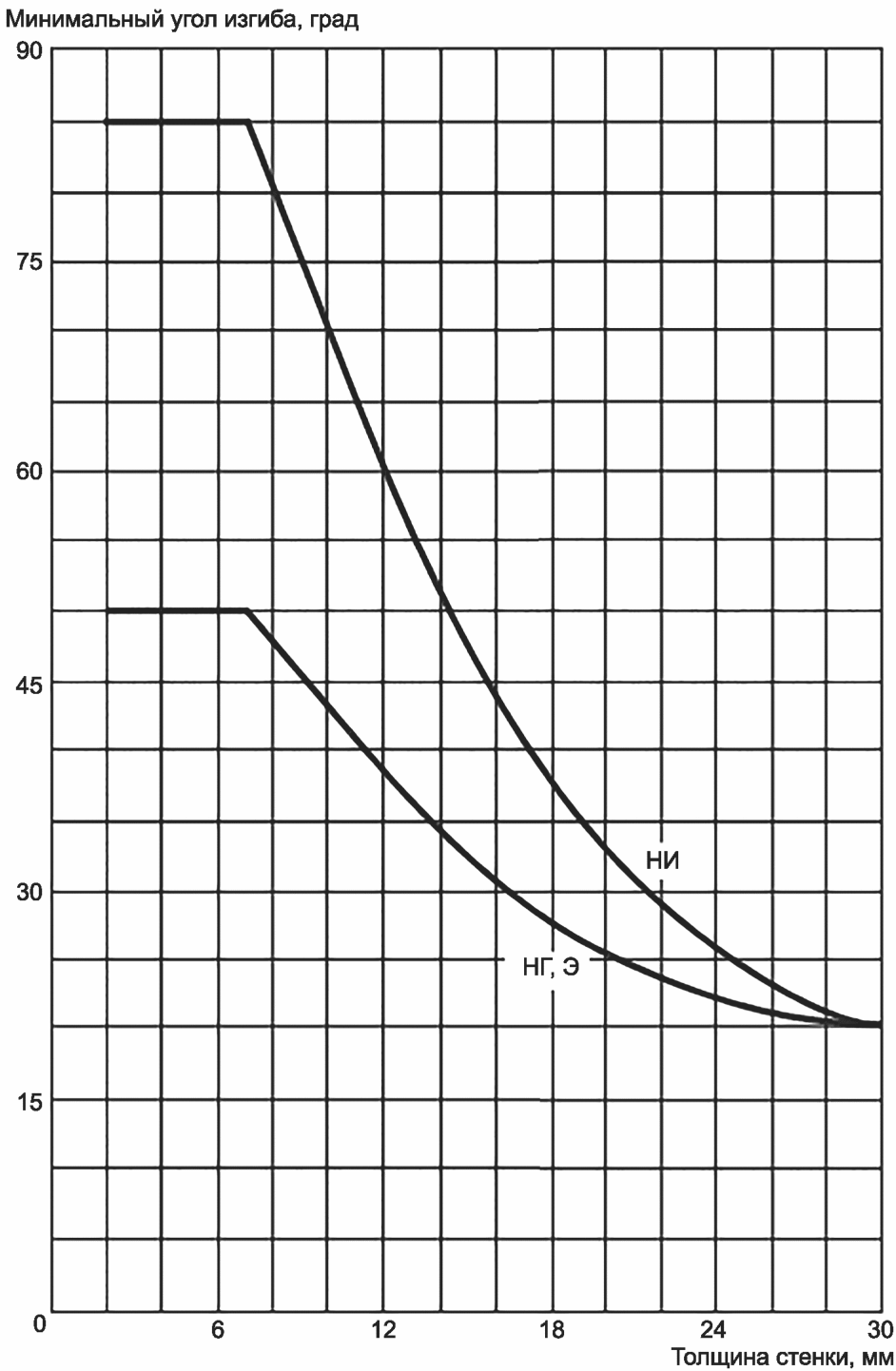
Рисунок Б.2 — Минимальный угол изгиба для ПП-В, ПП-Г и электропроводного ПЭ в зависимости от толщины для разных методов сварки (верхняя кривая — для сварки HI, нижняя — для сварки HG и Э)
