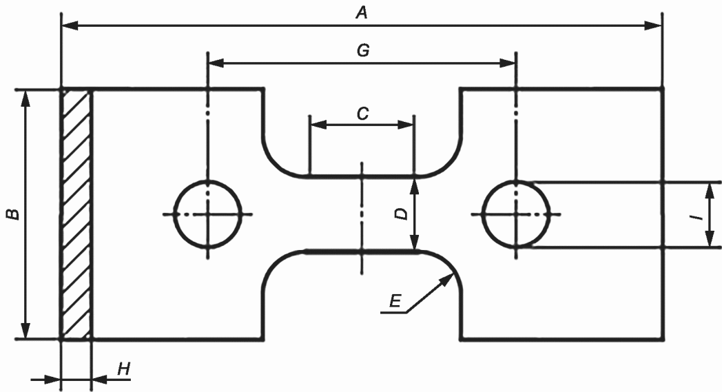
A — общая длина; B — ширина головки; C — длина узкой рабочей части; D — ширина узкой рабочей части; E — радиус; G — начальная длина между зажимами; H — толщина; I — диаметр отверстий для штифтов
